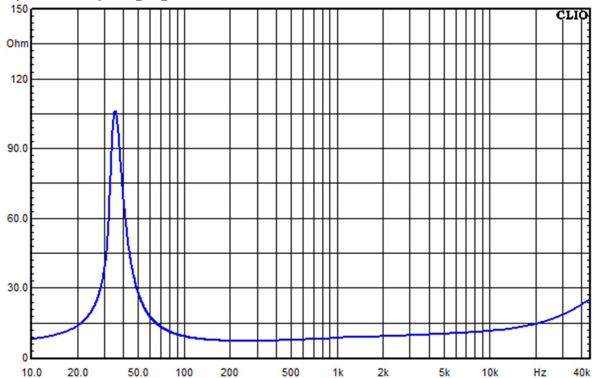
Abbildung 4: Wavecor WF182CU12-Impedanzverlauf
