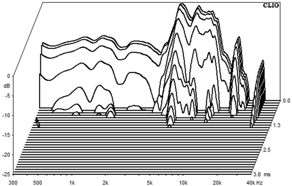
Abbildung 5: Wavecor WF182CU12-Wasserfallsspektrum auf Achse (0°)
