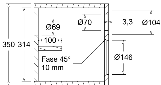
Schnitt A-A'
