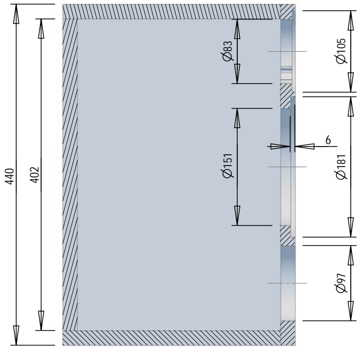
Schnitt A-A'
