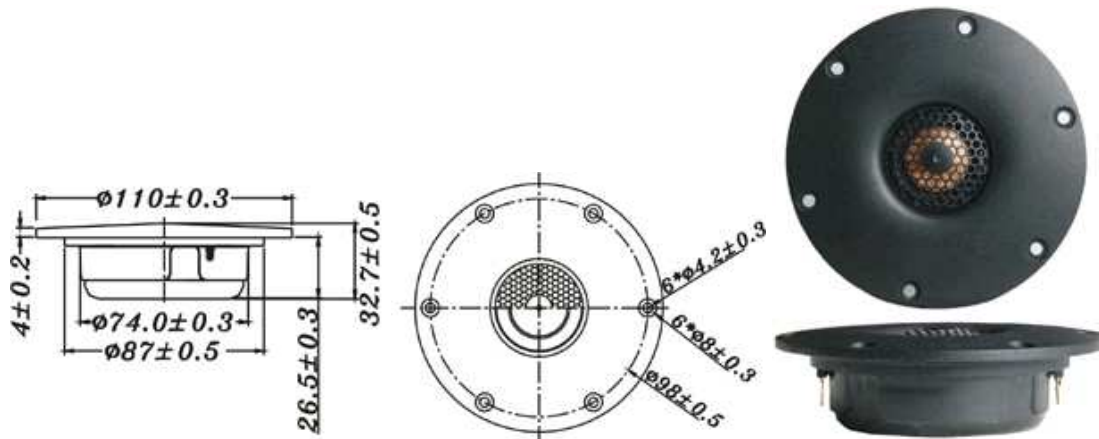
25mm BERYLLIUM DOME TWEETER
